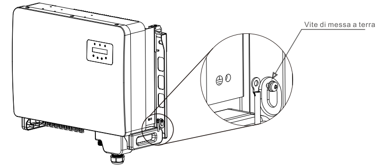
Figura 5.9 Cavo fissato
