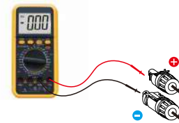
Figura 5.16 Misurazione con Multimetro
