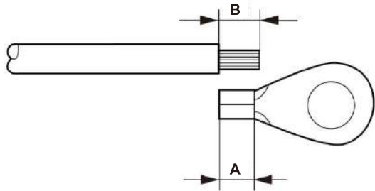
Figura 5.7 Lunghezza idonea
