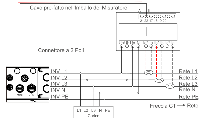
Figura 5.27 Misuratore di CT Esterno - "Misuratore in Rete"
