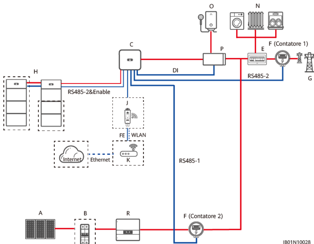
Figura 3-18 Connessione in rete con inverter di terze parti
