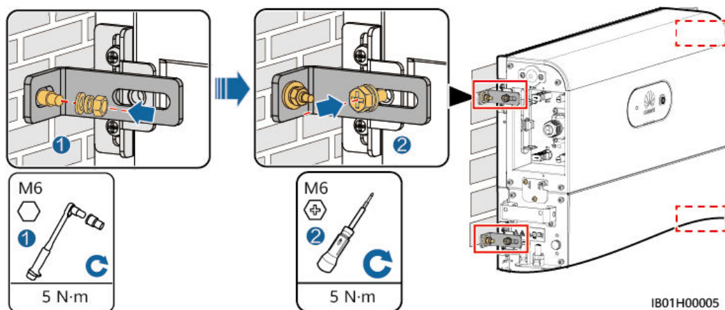
Figura 4-6 Fissaggio del modulo di controllo dell'alimentazione
