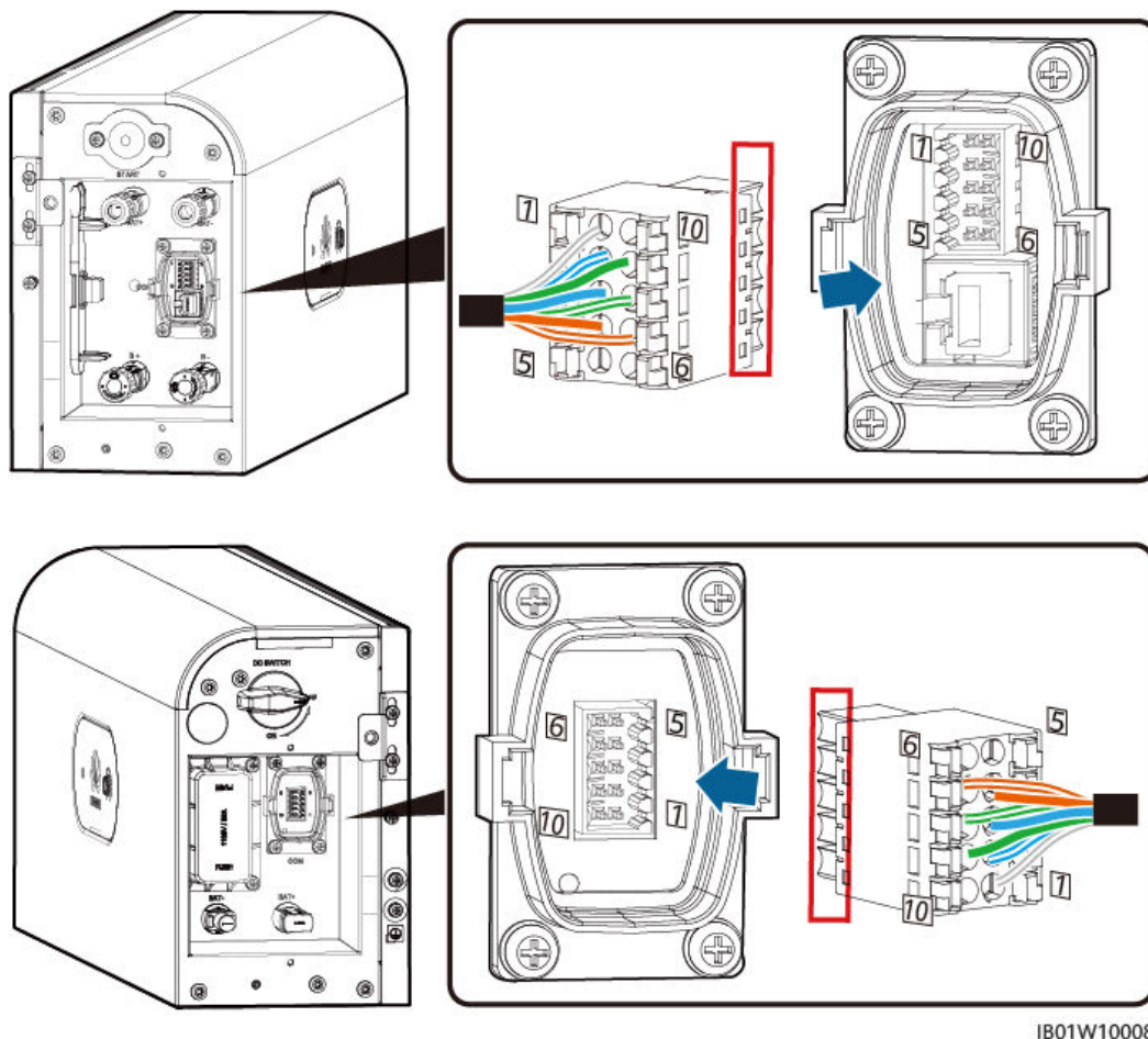
Figura 5-15 Inserimento del terminale
