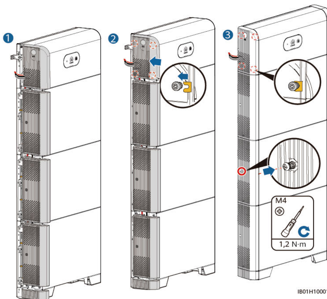
Figura 5-17 Installazione del coperchio
