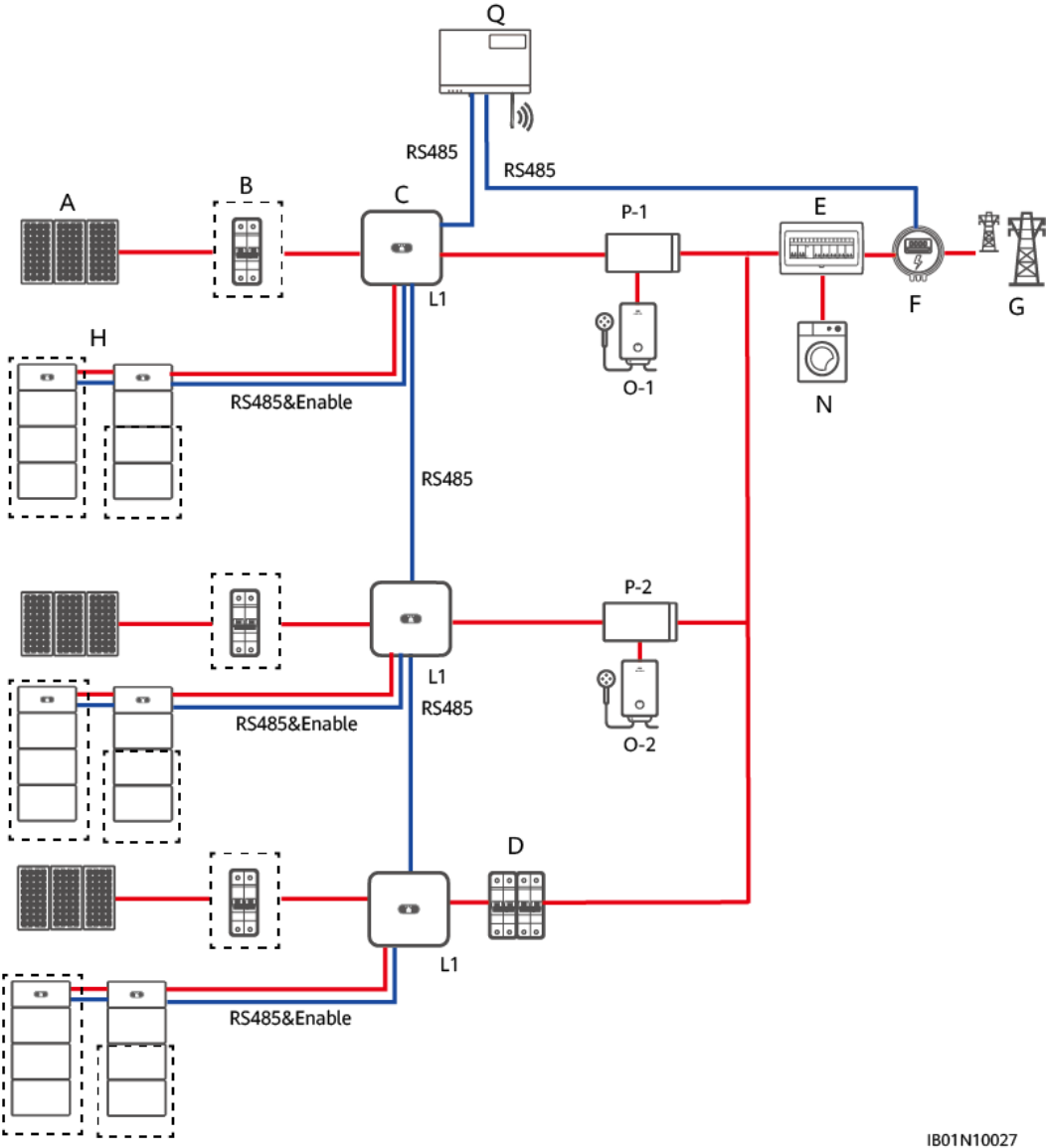
Figura 3-13 Diagramma di connessione di rete degli inverter SUN2000-(2KTL-6KTL)-L1 collegati in cascata (i riquadri tratteggiati indicano i componenti opzionali)
