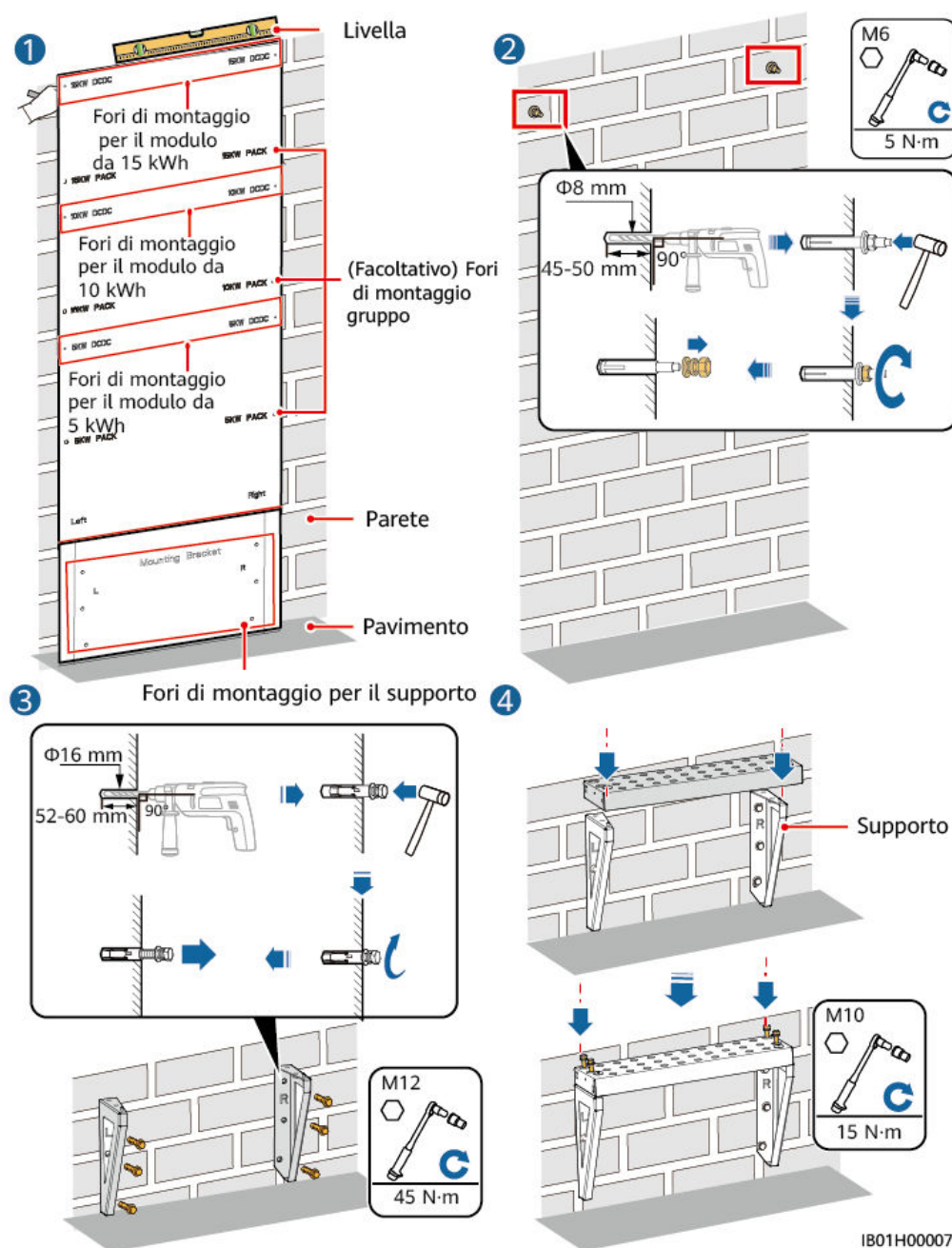
Figura 4-8 Installazione a parete
