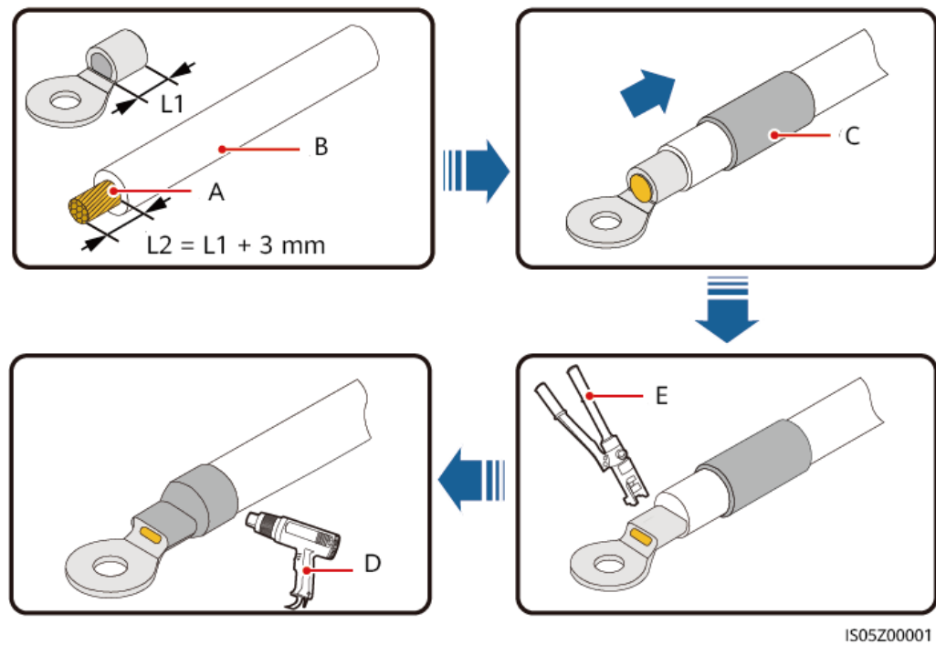
Figura 5-7 Crimpatura di un terminale OT
