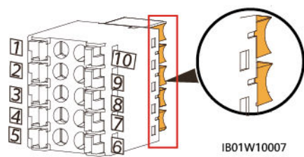
Figura 5-11 Porte dei cavi di segnale
