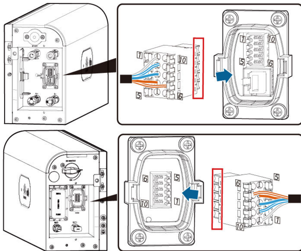
Figura 5-12 Inserimento del terminale
