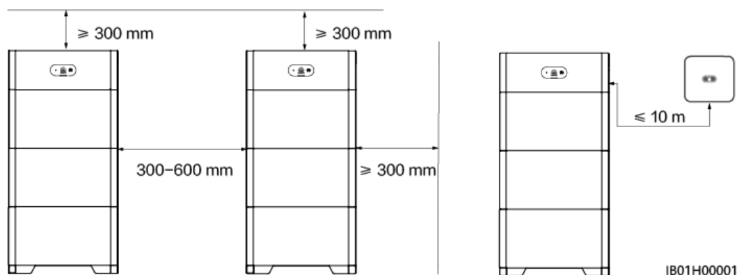
Figura 4-1 Spazio di installazione
