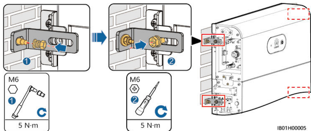
Figura 4-9 Fissaggio del modulo di controllo dell'alimentazione
