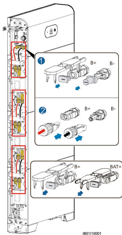
Figura 5-3 Collegamento del cavo di alimentazione CC all'interno della batteria
