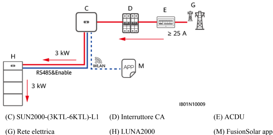
Figura 7-2 Diagramma di rete per uno scenario con alimentazione monofase
