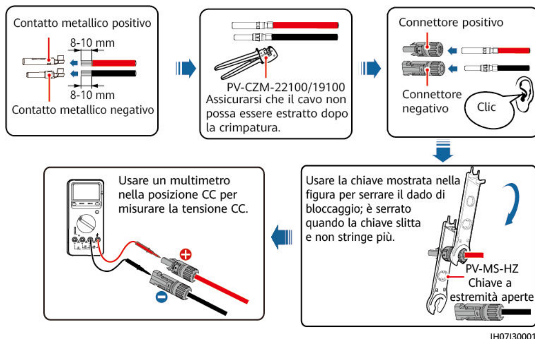
Figura 5-9 Assemblaggio dei connettori CC
