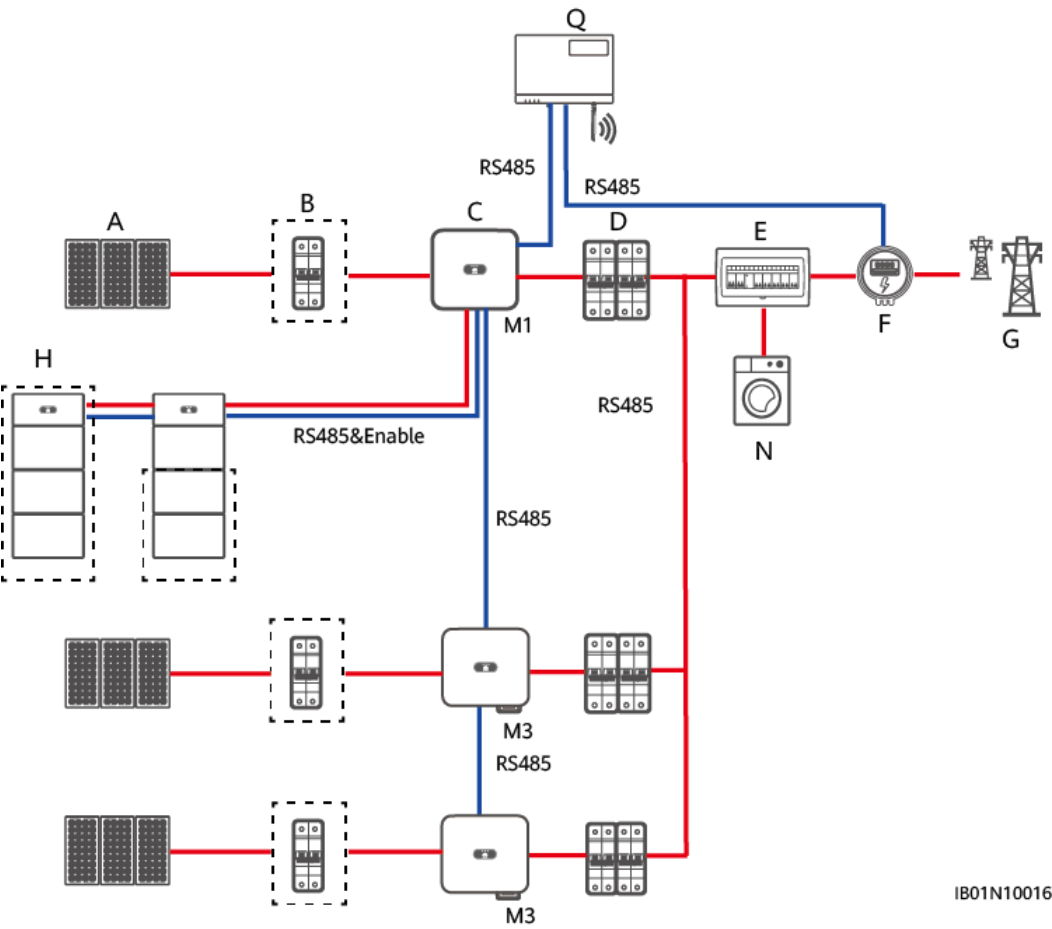
Figura 3-2 Collegamento in rete di un SUN2000-(3KTL-10KTL)-M1 e due SUN2000-(20KTL, 29.9KTL, 30KTL, 36KTL, 40KTL)-M3 (i riquadri tratteggiati indicano i componenti opzionali)
