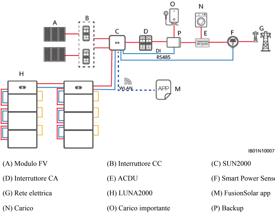
Figura 5-1 Collegamento dei cavi della batteria
