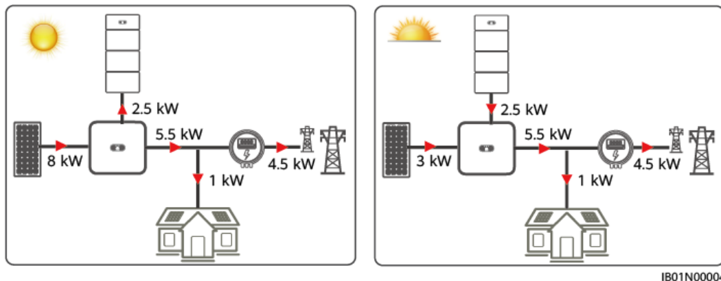
Figura 3-10 Esempio di modalità Inviata integralmente alla rete
