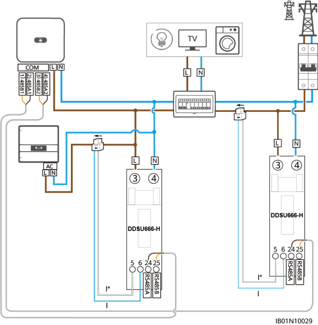
Figura 3-19 Collegamenti dei cavi del contatore elettrico per SUN2000-(2KTL-6KTL)-L1
