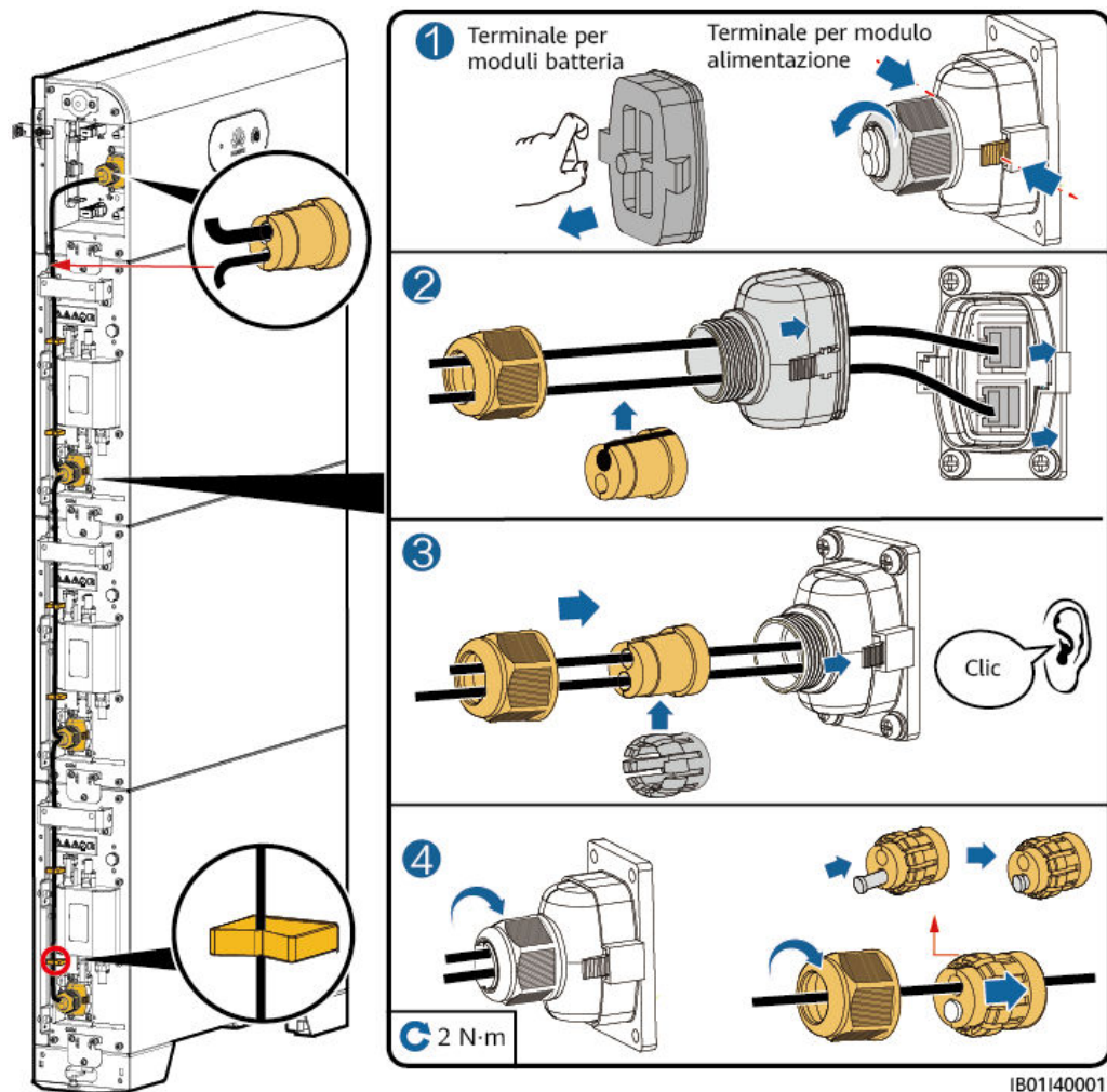
Figura 5-4 Fissaggio con le clip
