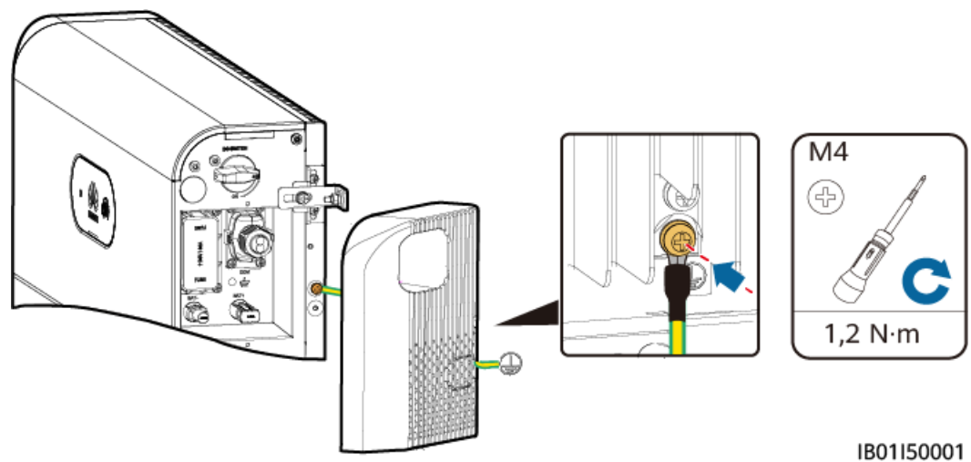
Figura 5-8 Messa a terra del cavo PE
