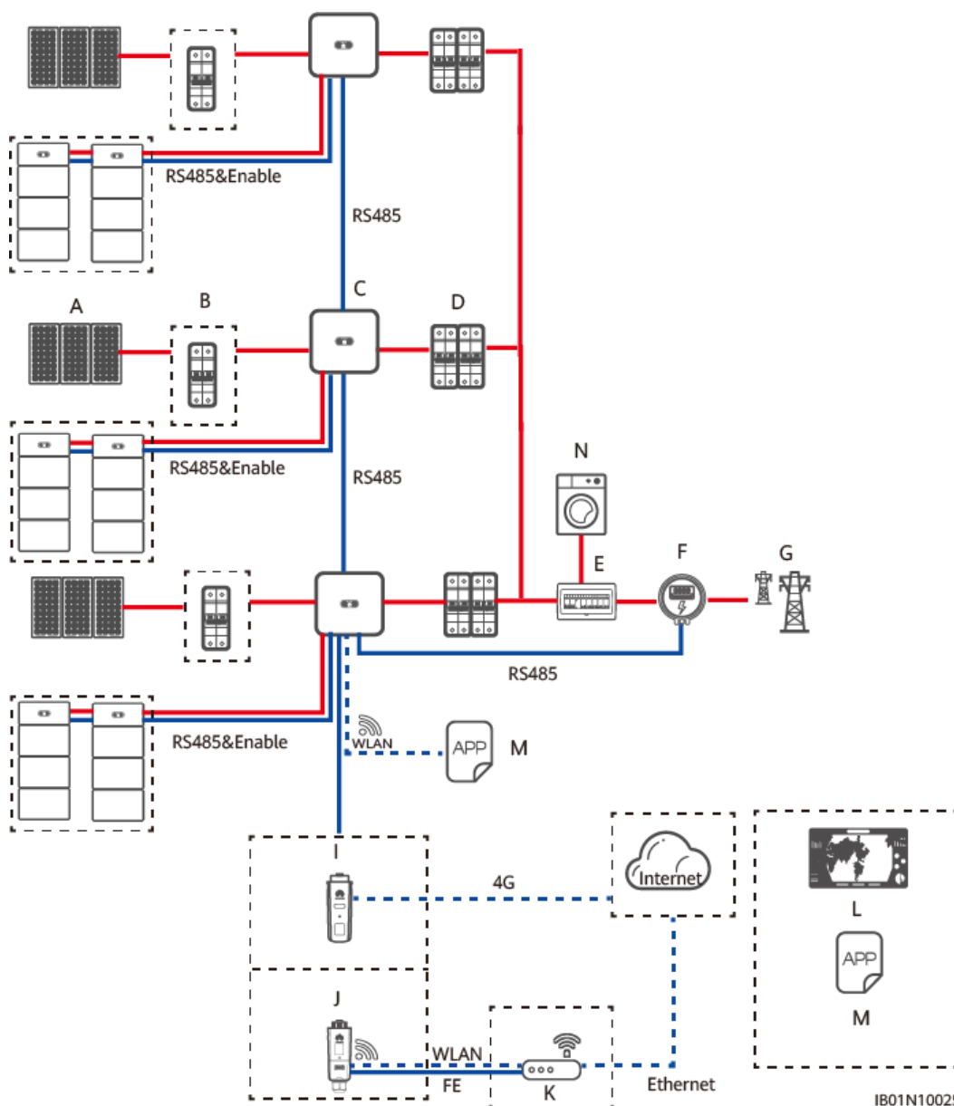
Figura 3-4 Connessione in rete dello Smart Dongle (i riquadri tratteggiati indicano i componenti opzionali)
