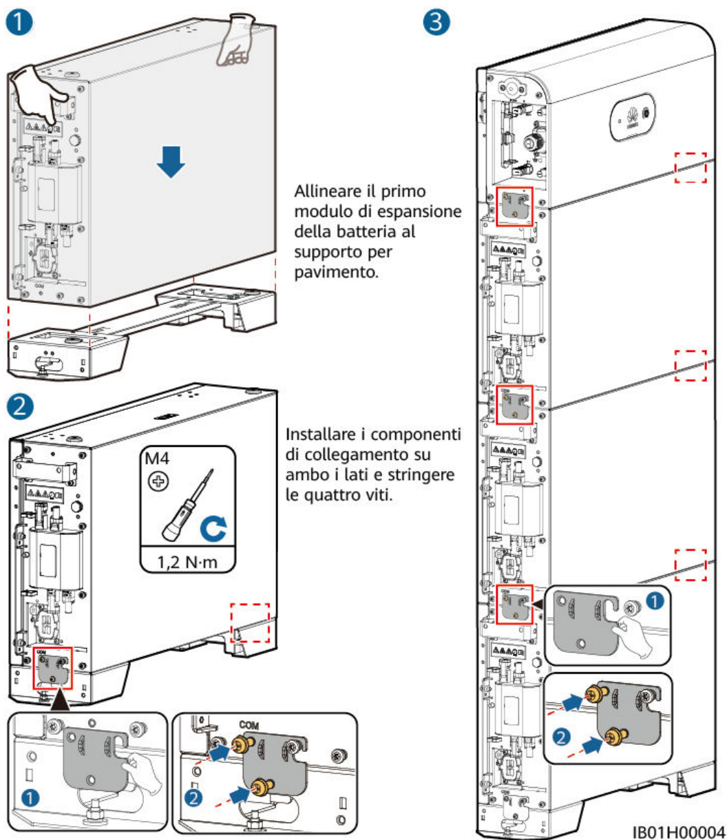
Figura 4-5 Installazione dei moduli di espansione della batteria e del modulo di controllo dell'alimentazione
