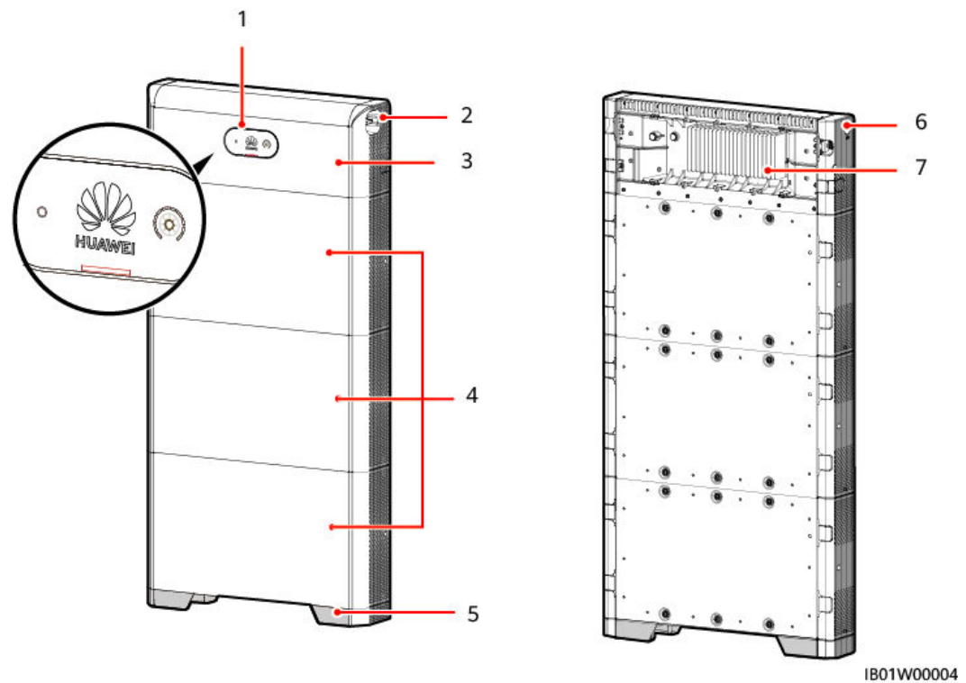
Figura 2-6 Aspetto della batteria
