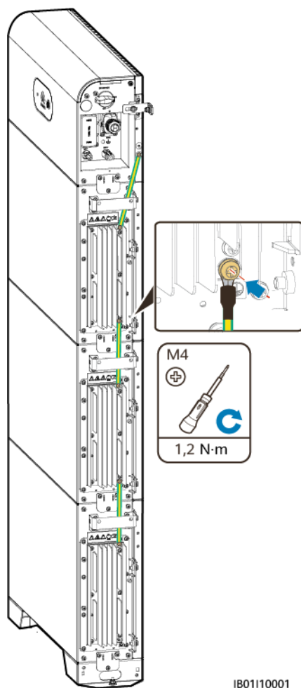
Figura 5-2 Collegamento del cavo PE interno
