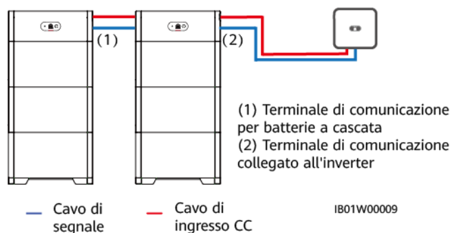
Figura 5-14 Connessione dei cavi per collegamento in cascata delle batterie
