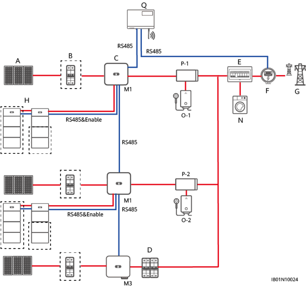
Figura 3-12 Connessione in rete di due SUN2000-(3KTL-10KTL)-M1 e un SUN2000-(20KTL, 29.9KTL, 30KTL, 36KTL, 40KTL)-M3 (i riquadri tratteggiati indicano i componenti opzionali)
