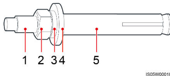
Figura 4-3 Schema della struttura di un bullone a espansione M6
