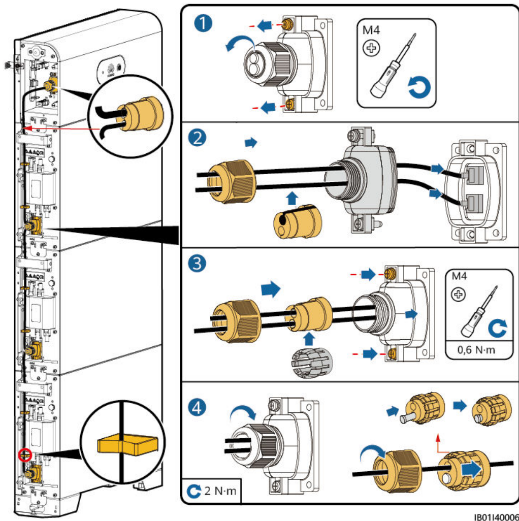
Figura 5-5 Fissaggio con le viti
