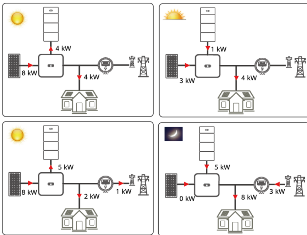
Figura 3-6 Esempio della modalità Energia autoconsumata
