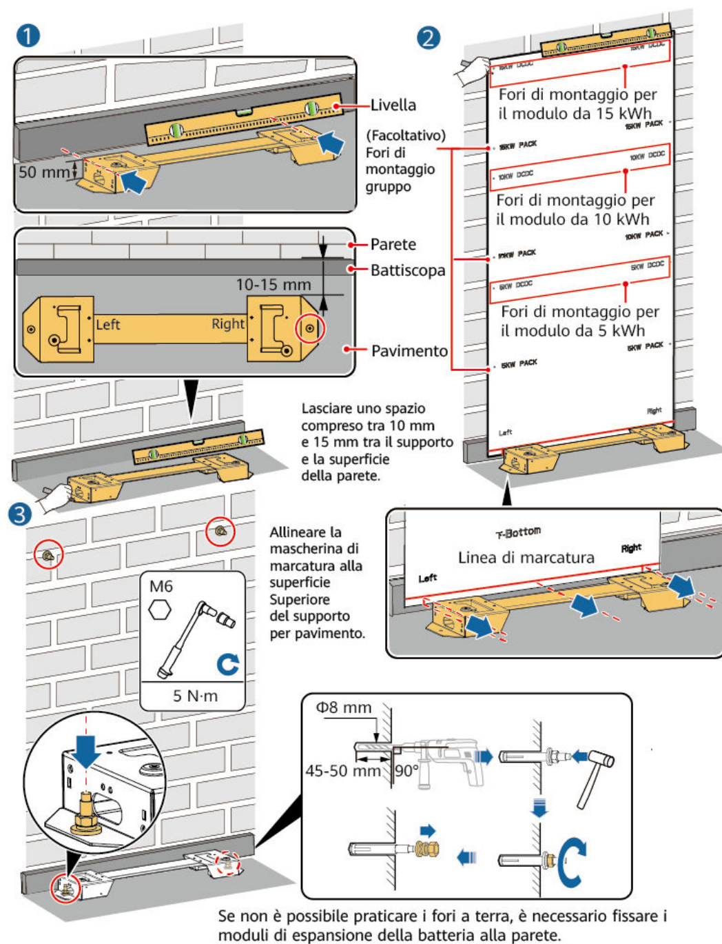
Figura 4-4 Installazione dei bulloni a espansione
