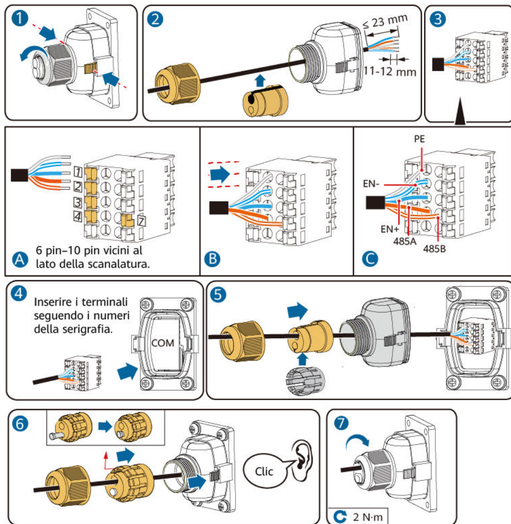
Figura 5-13 Collegamento dei terminali dell'inverter
