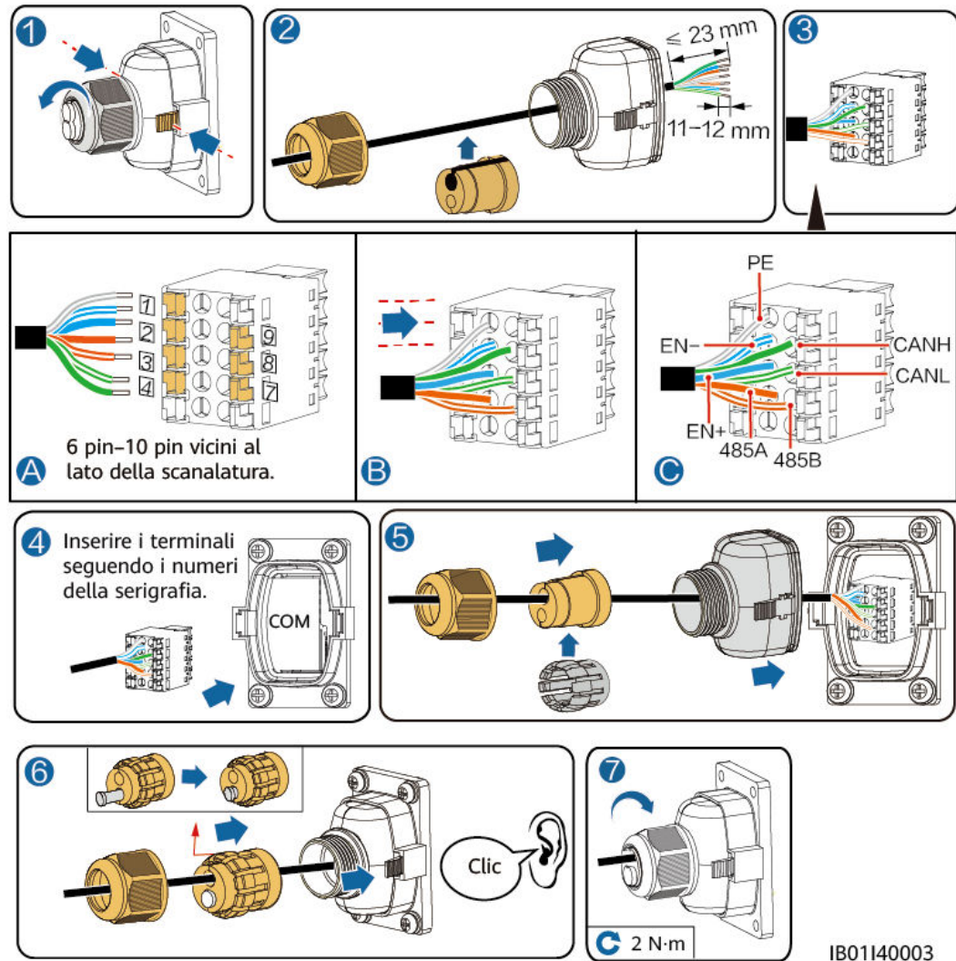
Figura 5-16 Terminale di comunicazione per collegamento in cascata
