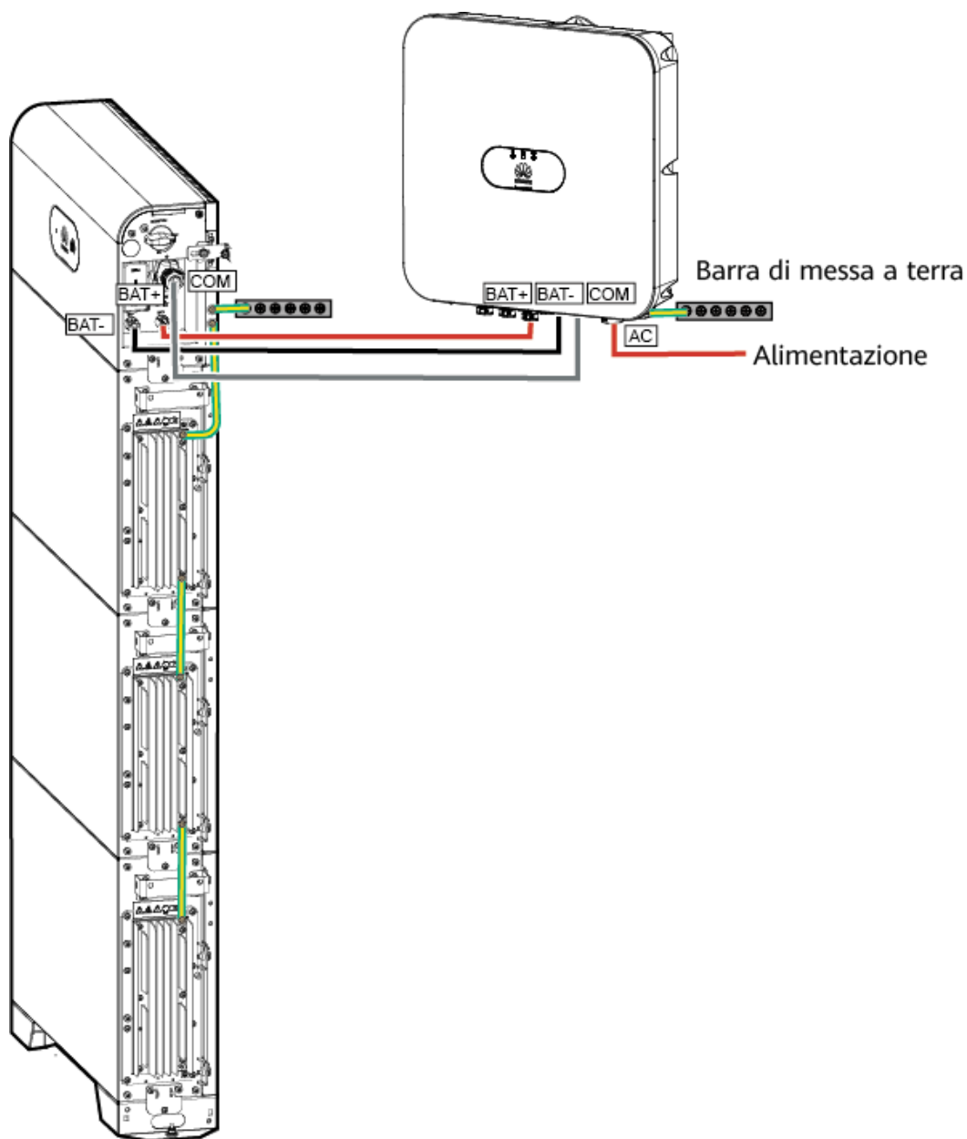
Figura 7-3 Schema di collegamento dei cavi
